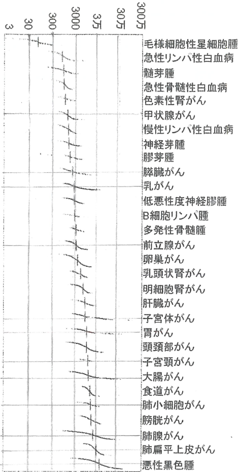
がん細胞1個当たりの変異数
